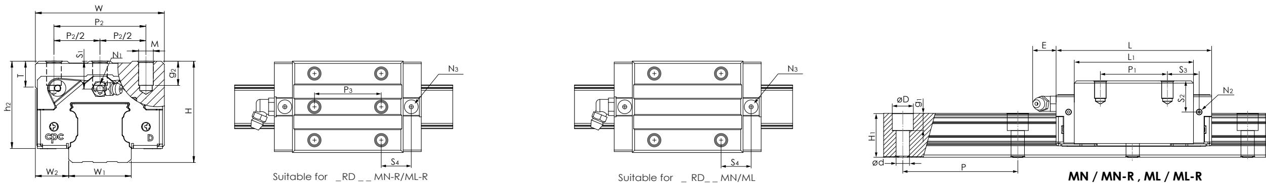
Dimensions Table
